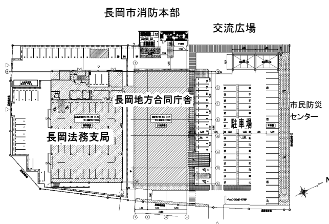
配置図
